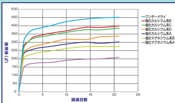
塩系乾燥剤 吸湿速度比較 25°C, RH90%強制循環
