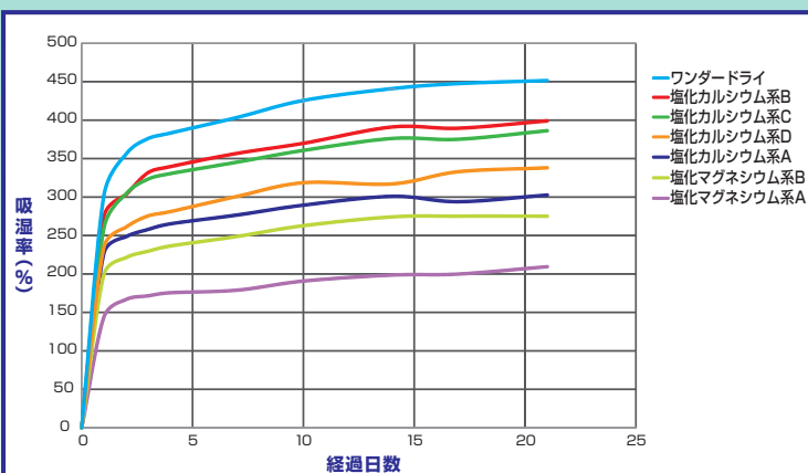
塩系乾燥剤 吸湿速度比較 25℃,RH90%強制循環
